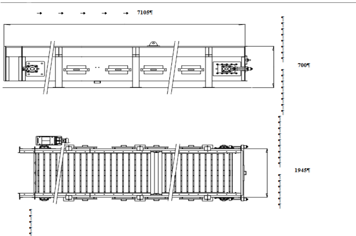
Foto 1 Nastro a piastre-tipologico
