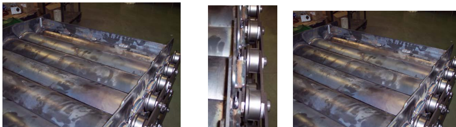
Foto 3 - Nastro a piastre tipo a tapparelle metalliche:
